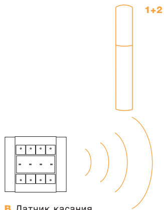
В Датчик касания, 4-секционный, со вставкой настенного радиопередатчика
